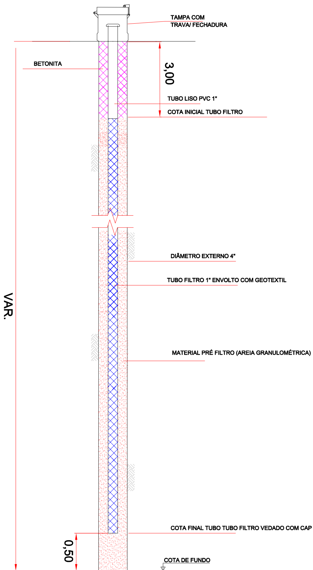
SEÇÃO ESQUEMÁTICA DO INDICADOR DE NÍVEL D'ÁGUA (INA) SEM ESCALA - MEDIDA EM METROS
