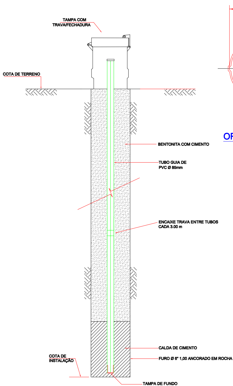
DETALHE ESQUEMÁTICO P/ INSTALAÇÃO DE INCLINÔMETRO (IN) SEM ESCALA - MEDIDA EM METROS
