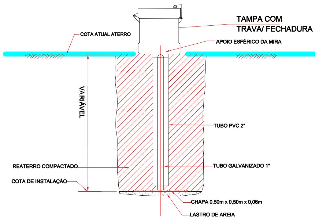
PLACA DE RECALQUE (PR) - PARA ATERRO SEM ESCALA
